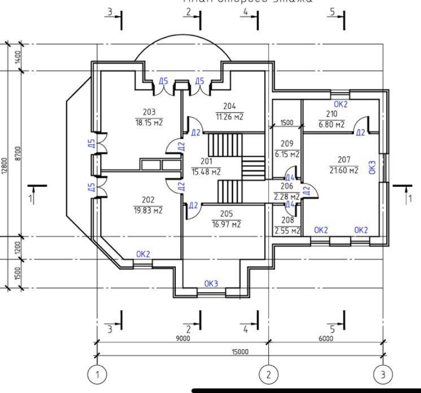
План второго этажа
